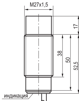
Габаритный чертеж
