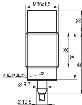
Габаритный чертеж
