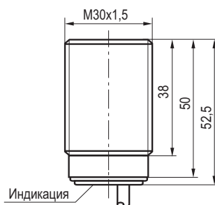
Габаритный чертеж
