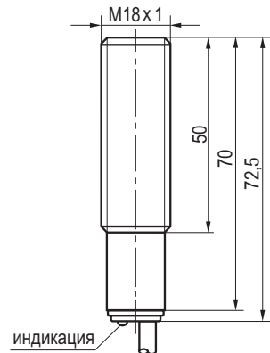
Габаритный чертеж
