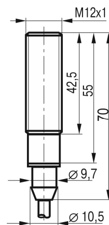
Габаритный чертеж
