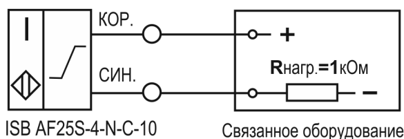
Схема подключения к оборудованию
