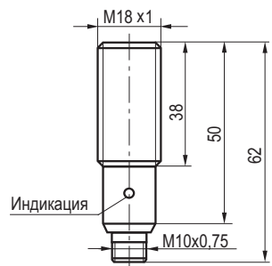
Габаритный чертеж
