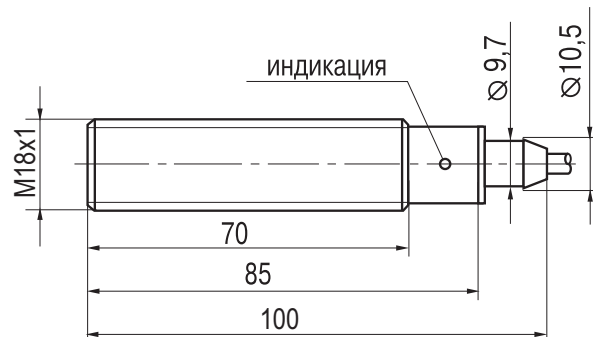
Габаритный чертеж
