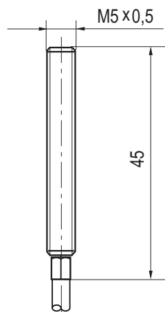
Габаритный чертеж
