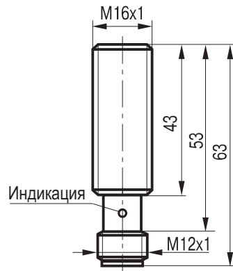
Габаритный чертеж
