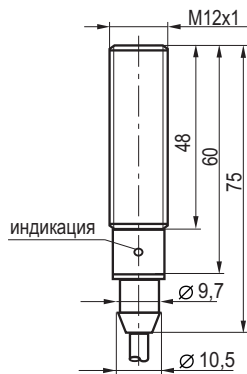
Габаритный чертеж
