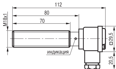
Габаритный чертеж
