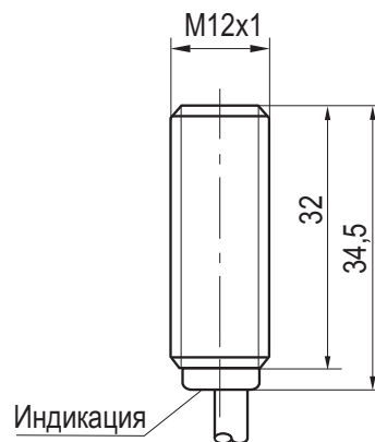
Габаритный чертеж
