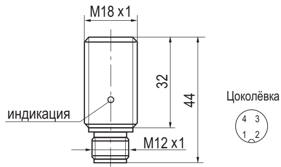
Габаритный чертеж
