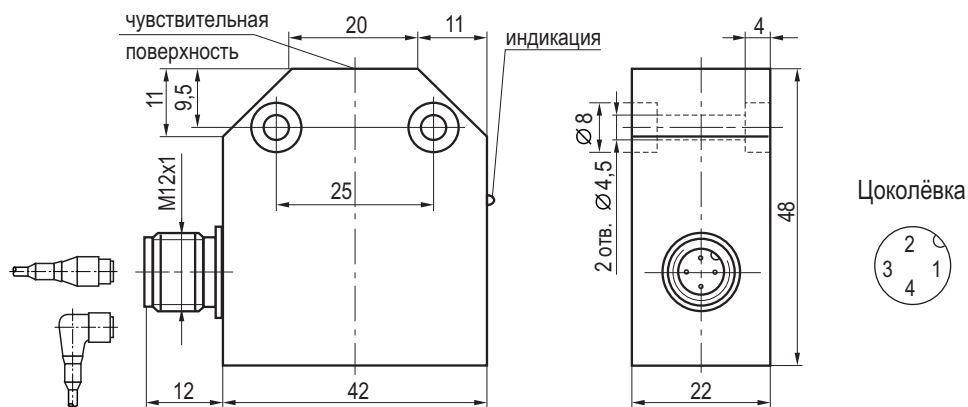
Габаритный чертеж
