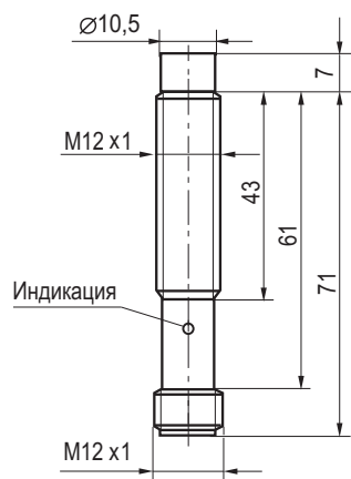
Габаритный чертеж
