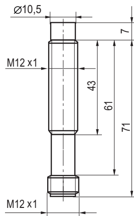
Габаритный чертеж
