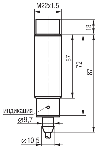
Габаритный чертеж
