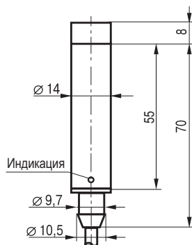
Габаритный чертеж
