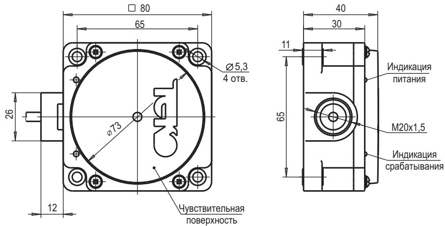
Габаритный чертеж
