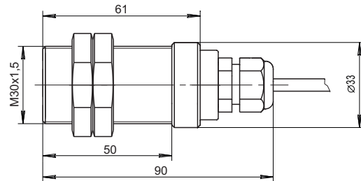
Габаритный чертеж
