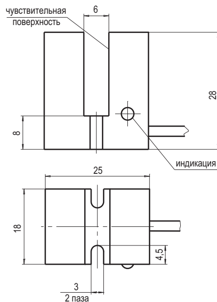
Габаритный чертеж
