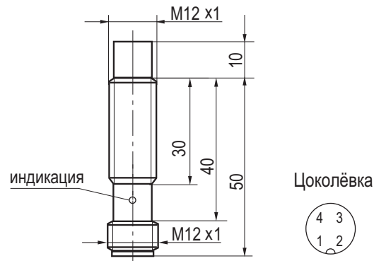
Габаритный чертеж
