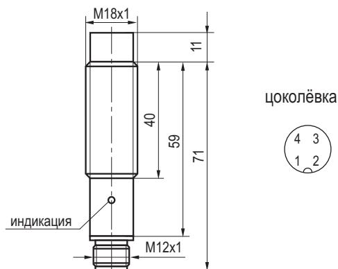
Габаритный чертеж
