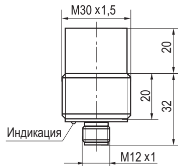
Габаритный чертёж
