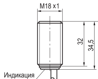
Габаритный чертеж
