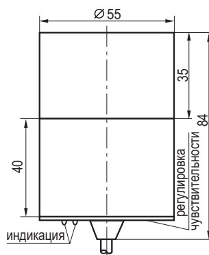
Габаритный чертеж
