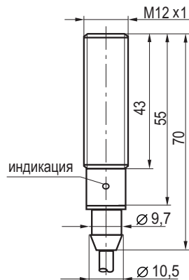
Габаритный чертеж
