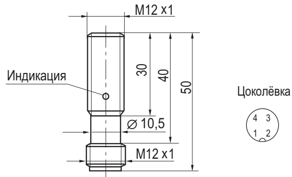
Габаритный чертеж
