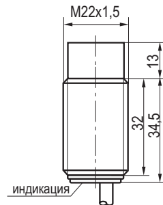
Габаритный чертеж
