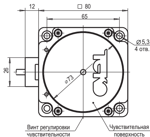
Габаритный чертеж
