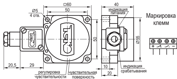
Габаритный чертеж
