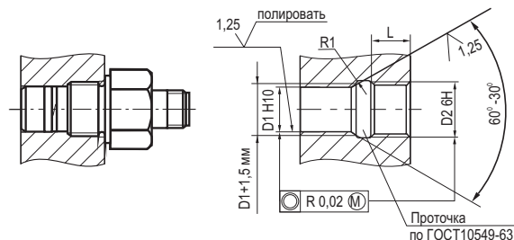
Схема монтажа
