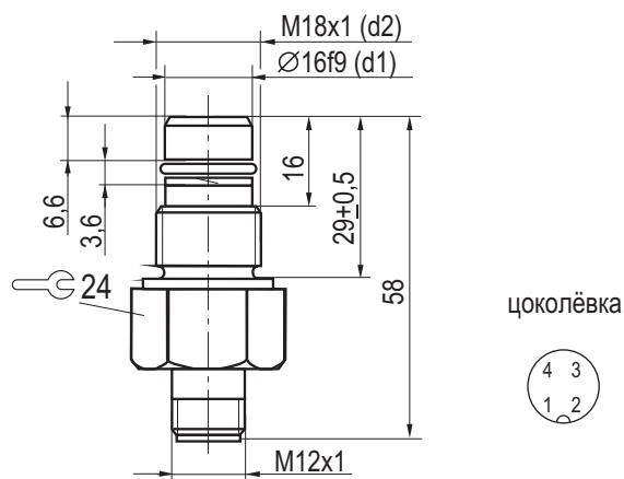
Габаритный чертеж
