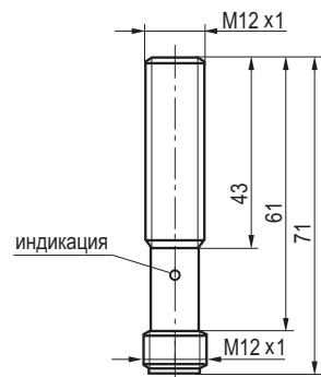
Габаритный чертеж
