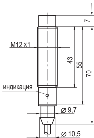
Габаритный чертеж
