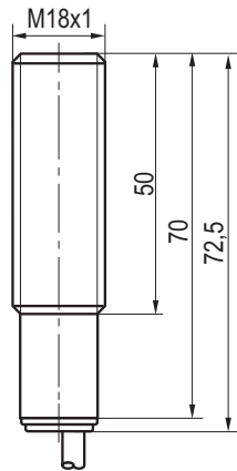
Габаритный чертеж
