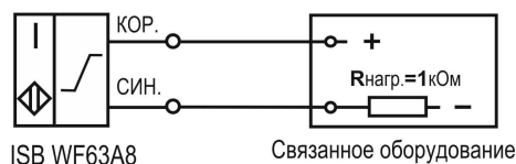
Схема подключения к оборудованию
