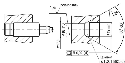
Схема монтажа
