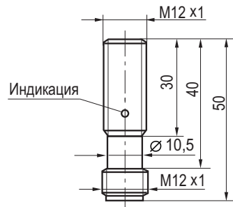
Габаритный чертеж
