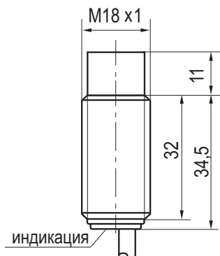
Габаритный чертеж
