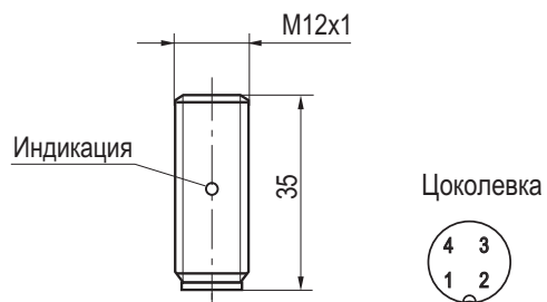
Габаритный чертеж
