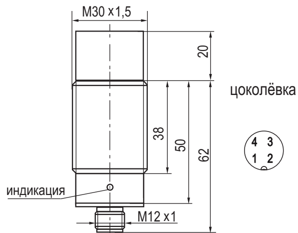
Габаритный чертеж
