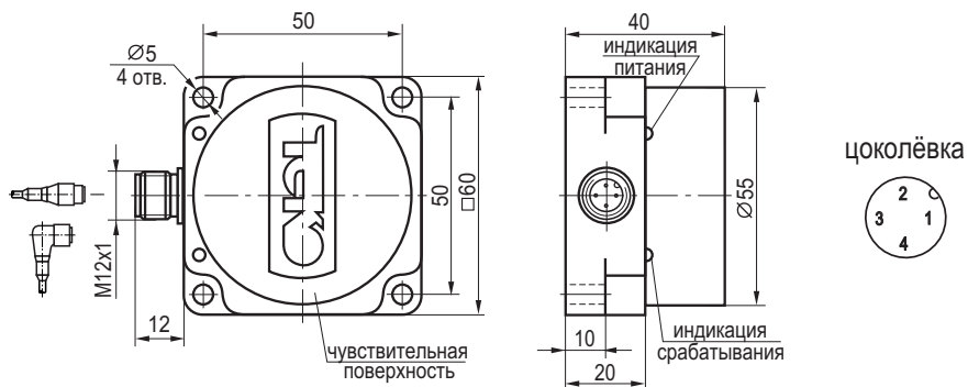
Габаритный чертеж
