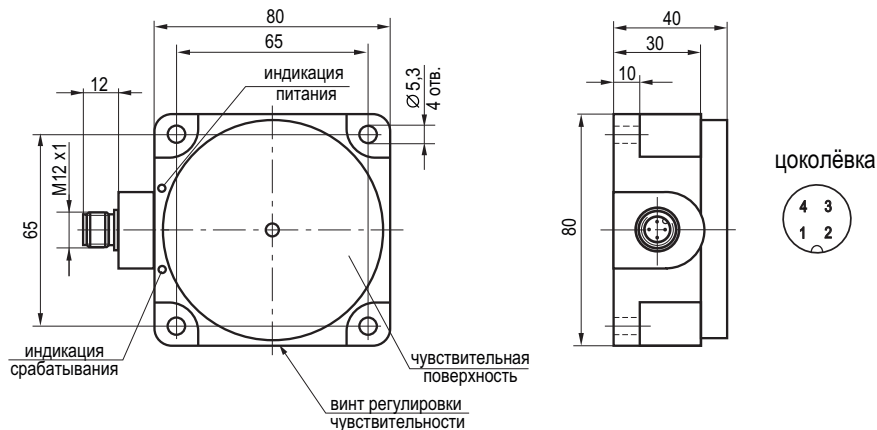
Габаритный чертеж
