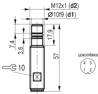
Габаритный чертеж
