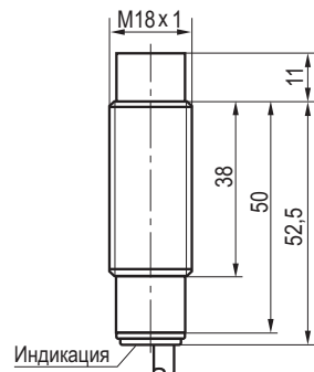
Габаритный чертеж
