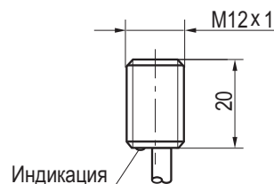
Габаритный чертеж
