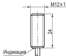
Габаритный чертеж
