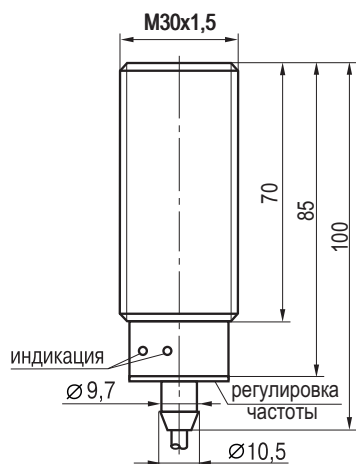
Габаритный чертеж
