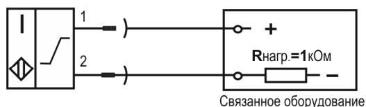
Схема подключения
