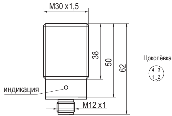
Габаритный чертеж
