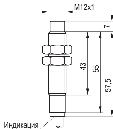
Габаритный чертеж
